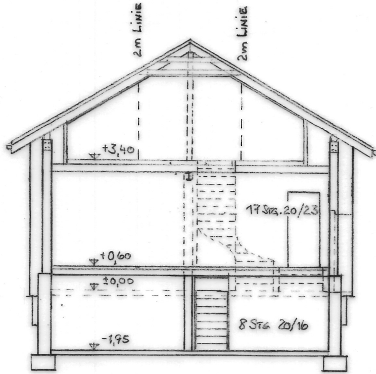
SCHNITT
