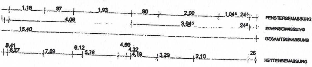
GRUNDRISS 106
