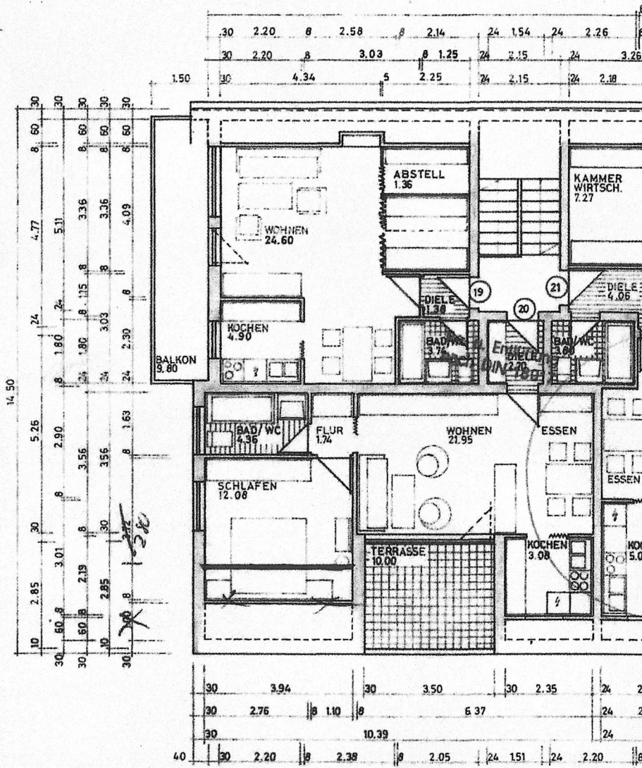
DACHGESCHOSS
