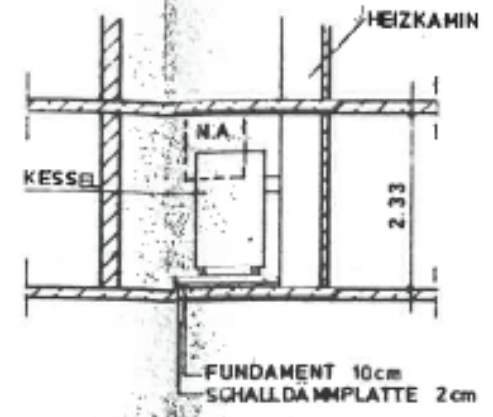
SCHNITT X - X
