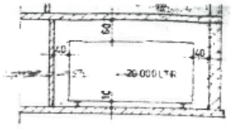
SCHNITT Y - Y (TANKR)
