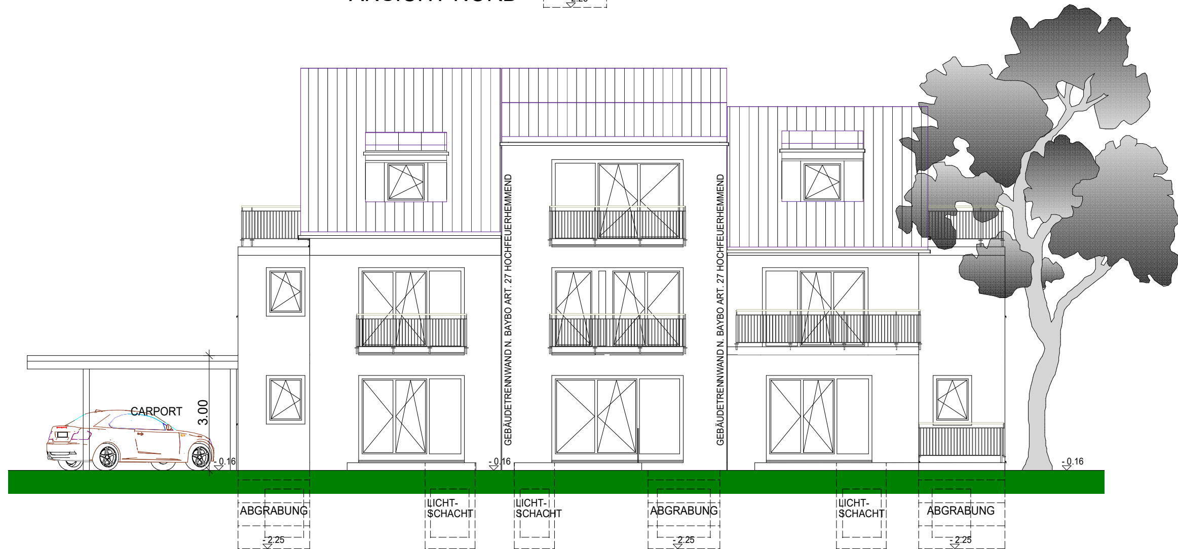
ANSICHT WEST
