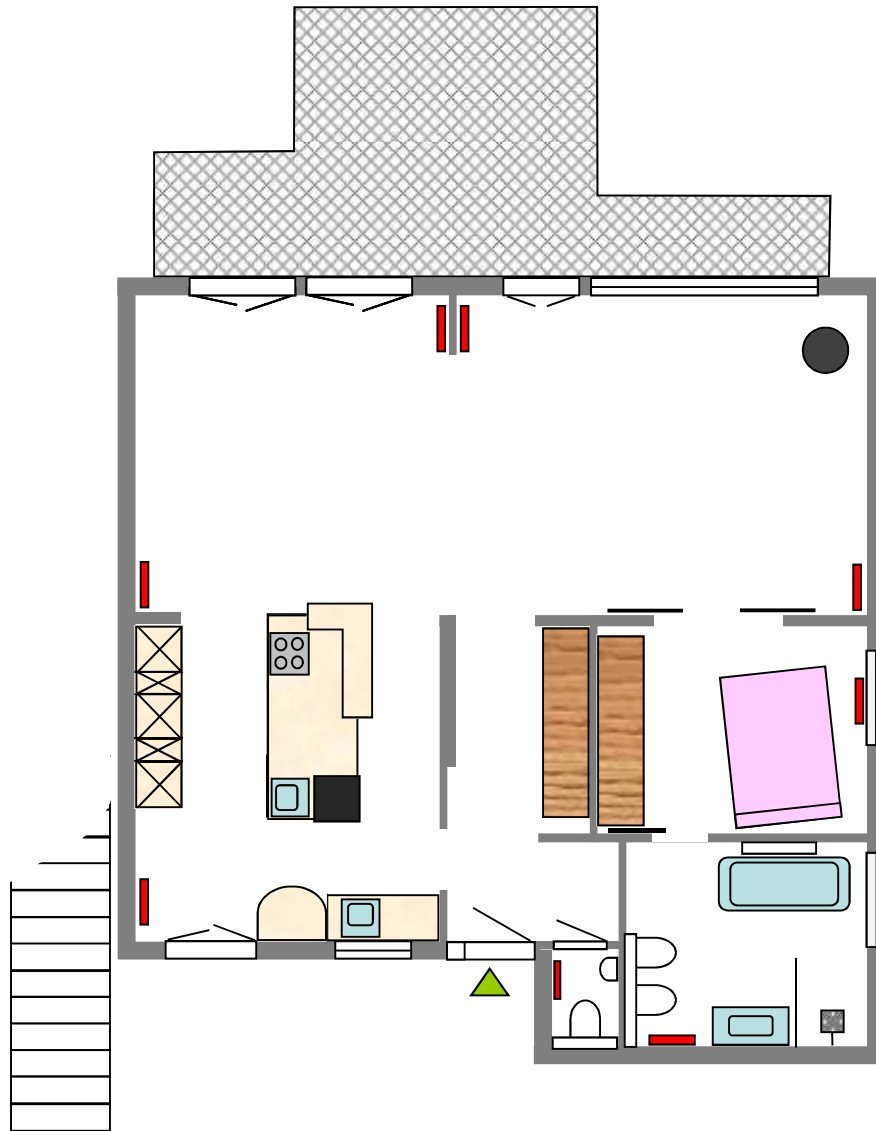
Grundriss Obergeschoss mit Balkon
