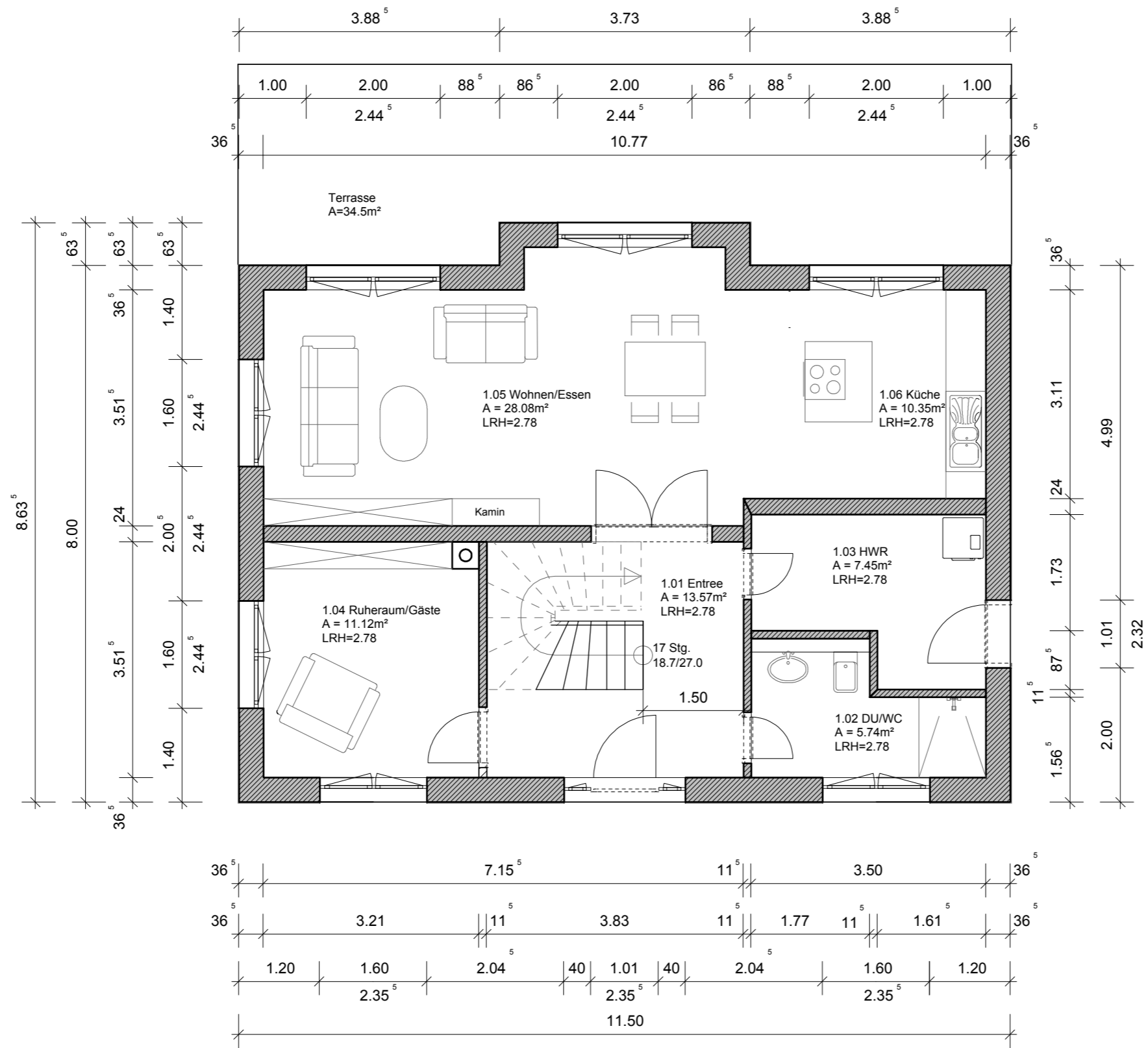
Grundriss Erdgeschoss
