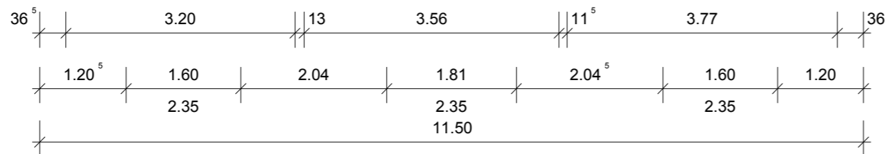
Grundriss Obergeschoss
