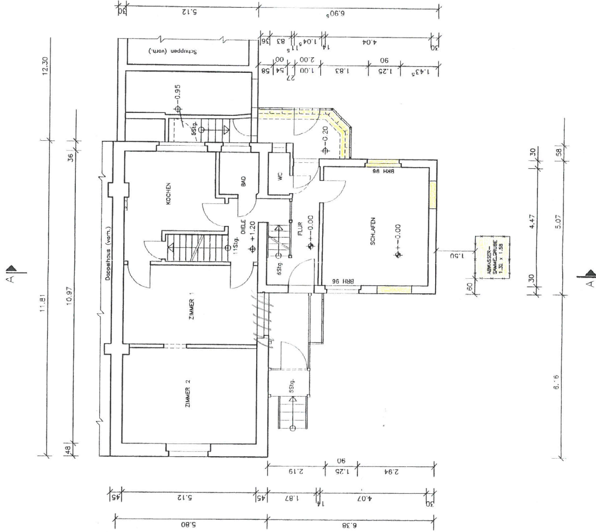
GRUNDRISS ERDGESCHOSS
