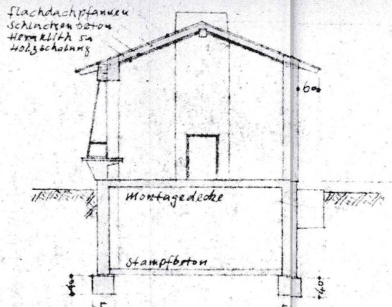
Schnitt B-B
