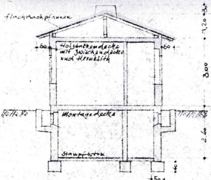
Schnitt A-A
