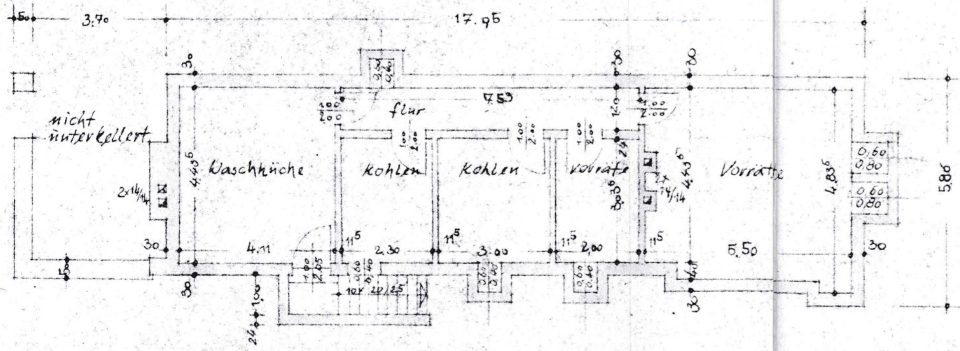
Kellergeschoss
