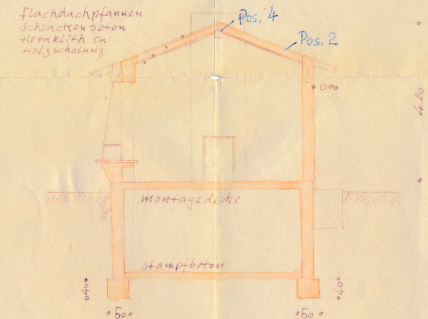
Schnitt B-B
