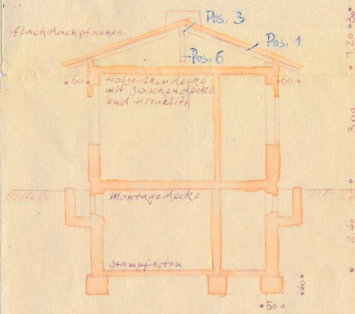
Schnitt A-A
