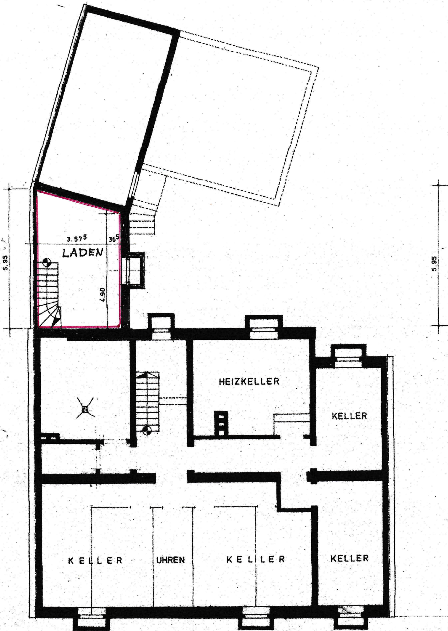
KELLERGESCHOSS
