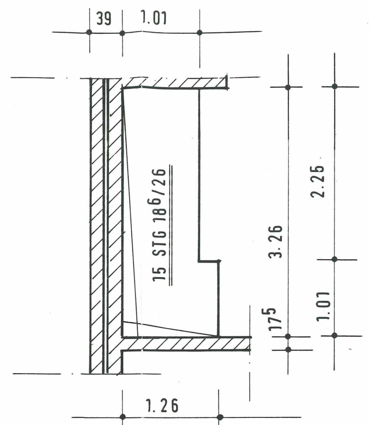
TREPPENLOCH EG 1 : 50
