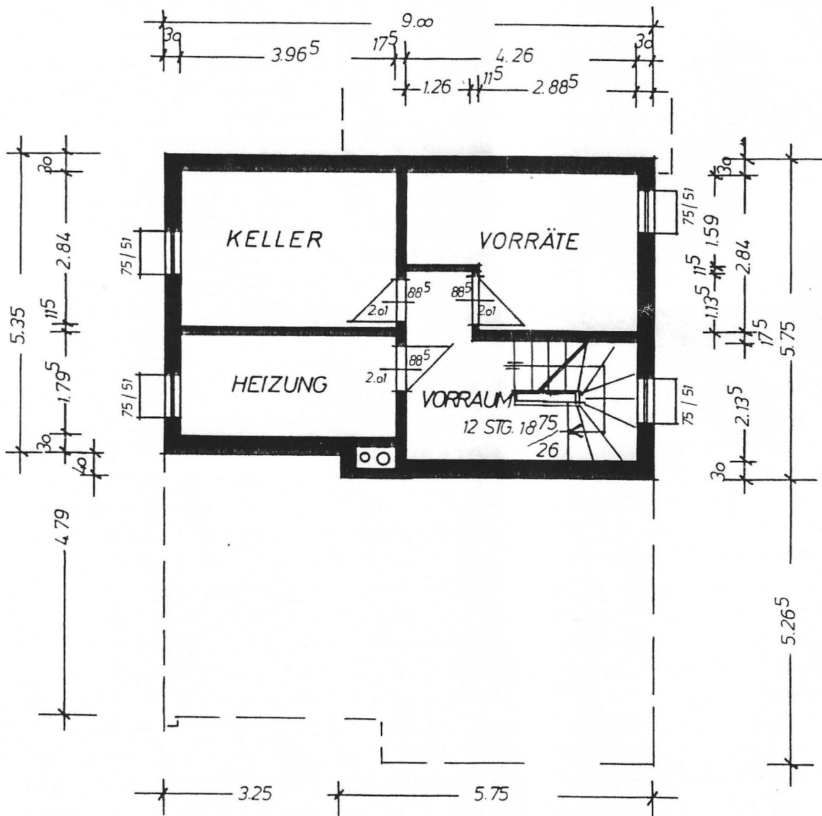
KELLERGESCHOSS
