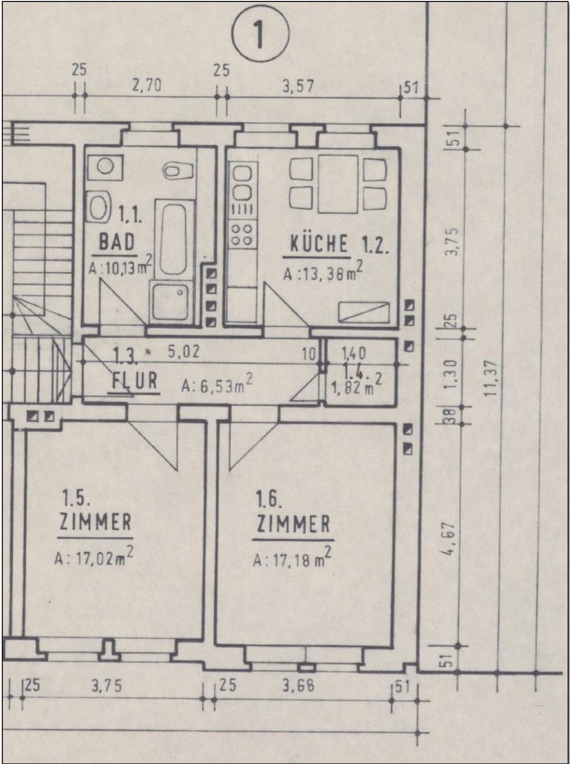
Grundriss Wohnung 1, Schopenhauerstraße 5 in 39108 Magdeburg
