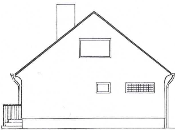
NORD - STRASSEN - ANSICHT
