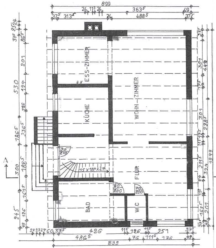
ERD - GESCHOSS
