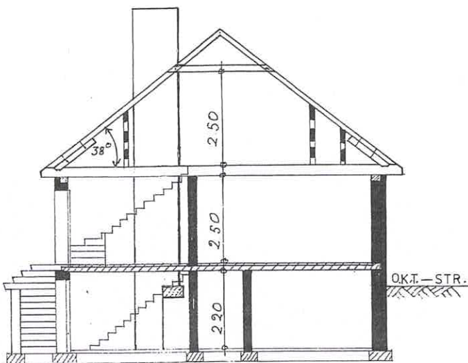
SCHNITT A-B
