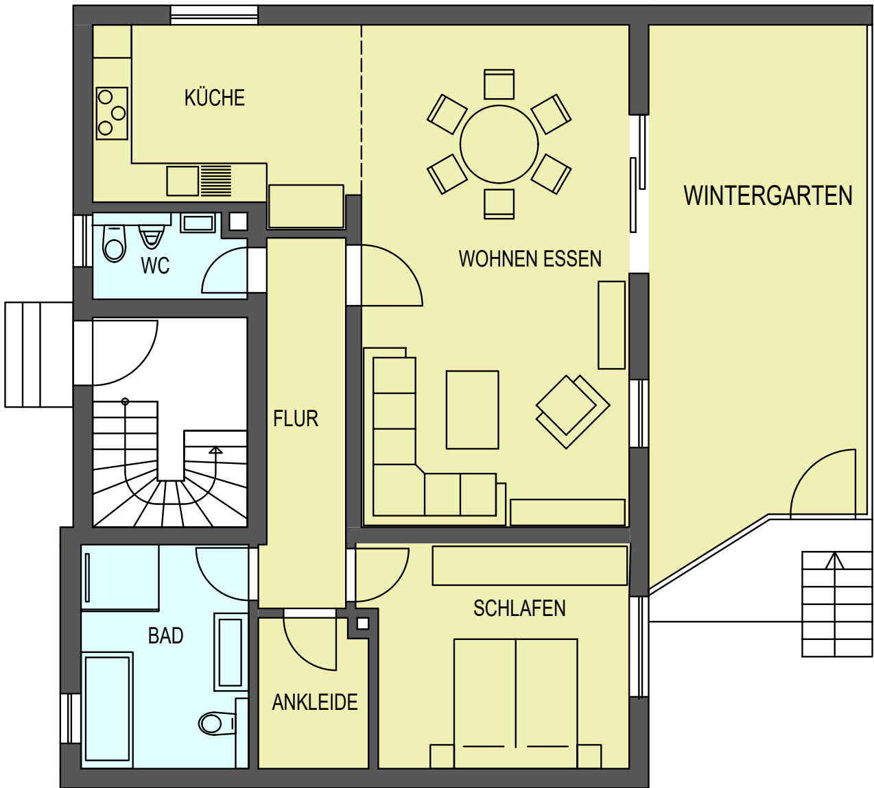
ERDGESCHOSS
