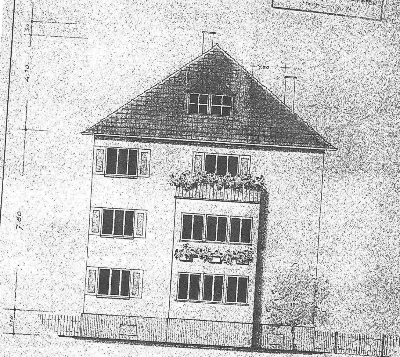
ANSICHT VON OSTEN M. 1:100
