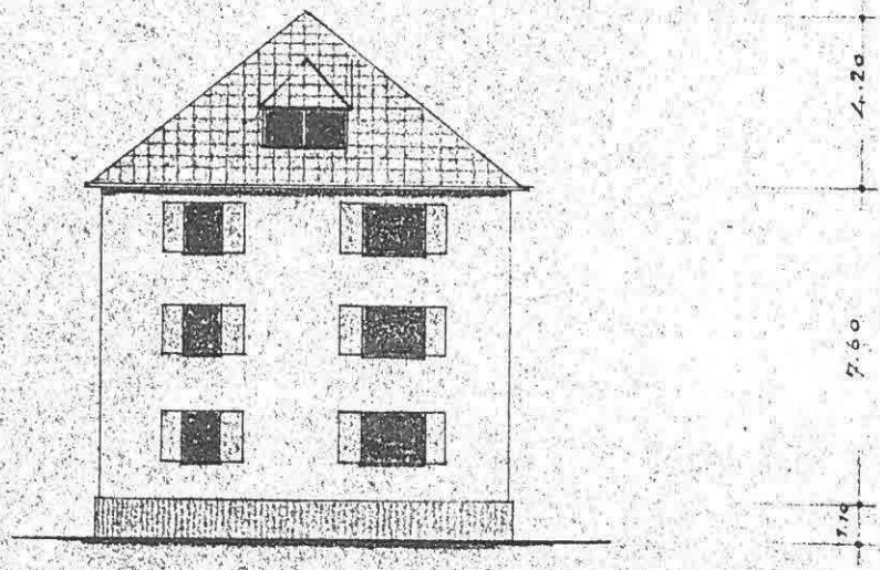
ANSICHT DER WESTSEITE M. 1:200
