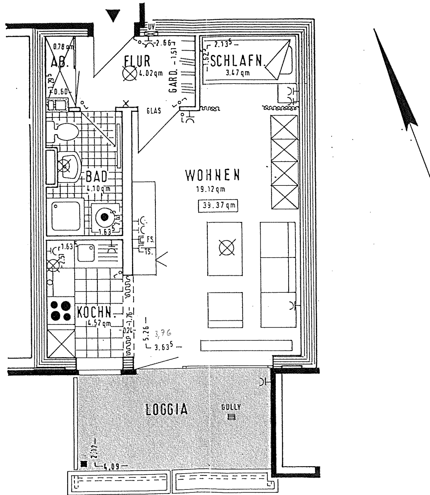
GRUNDRISS WOHNUNG NR. 2, 6, 10 u. 14
