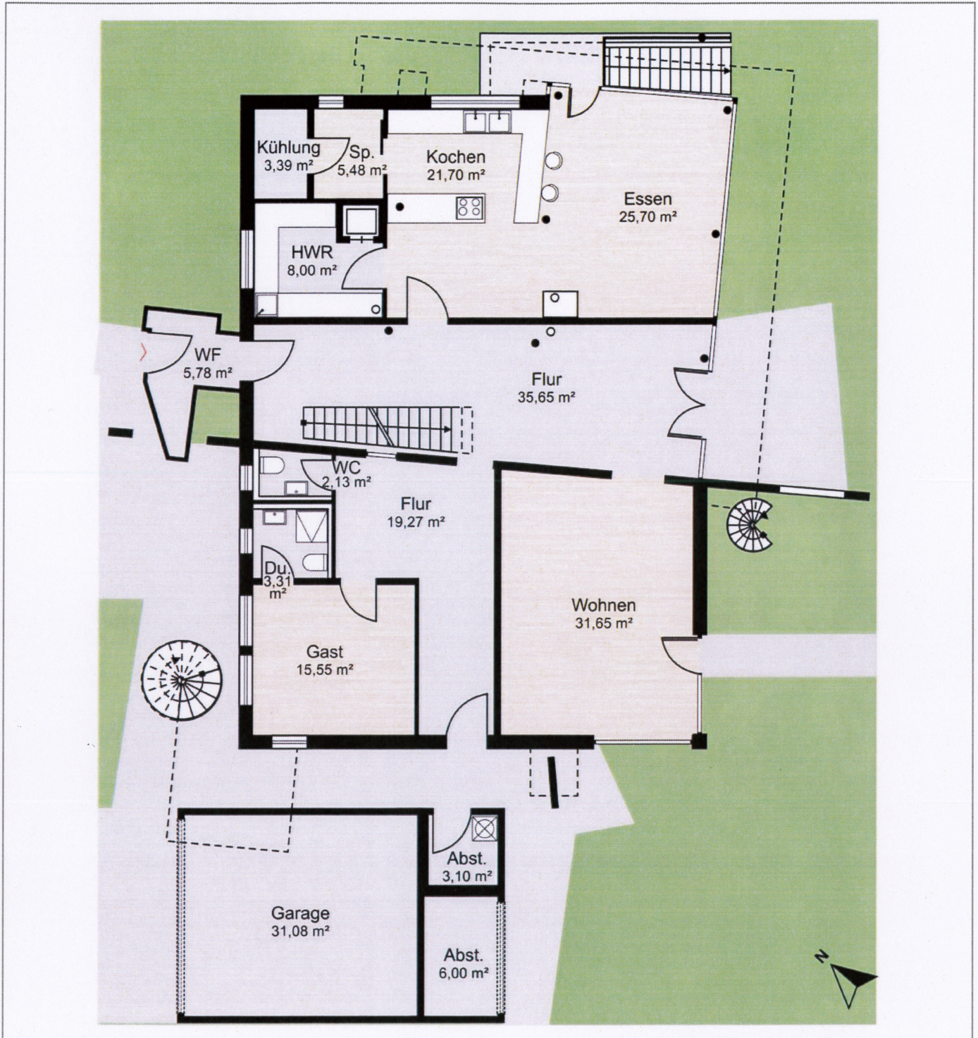
Grundriss Erdgeschoss
