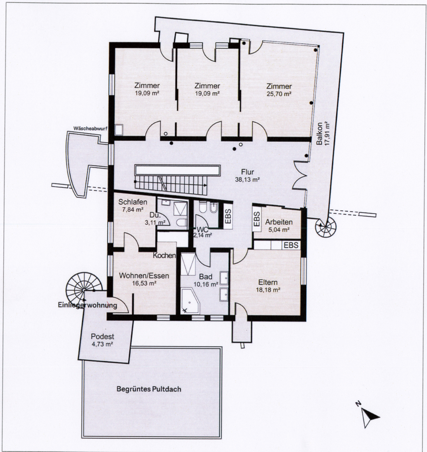
Grundriss Obergeschoss
