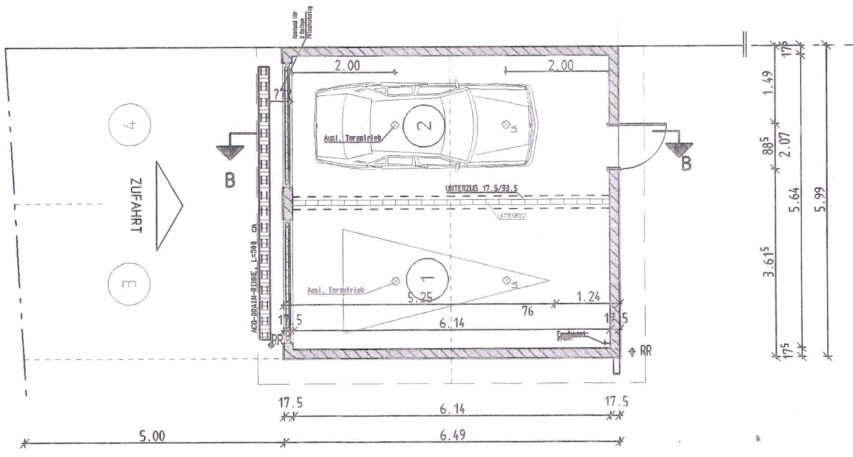
GRUNDRISS
