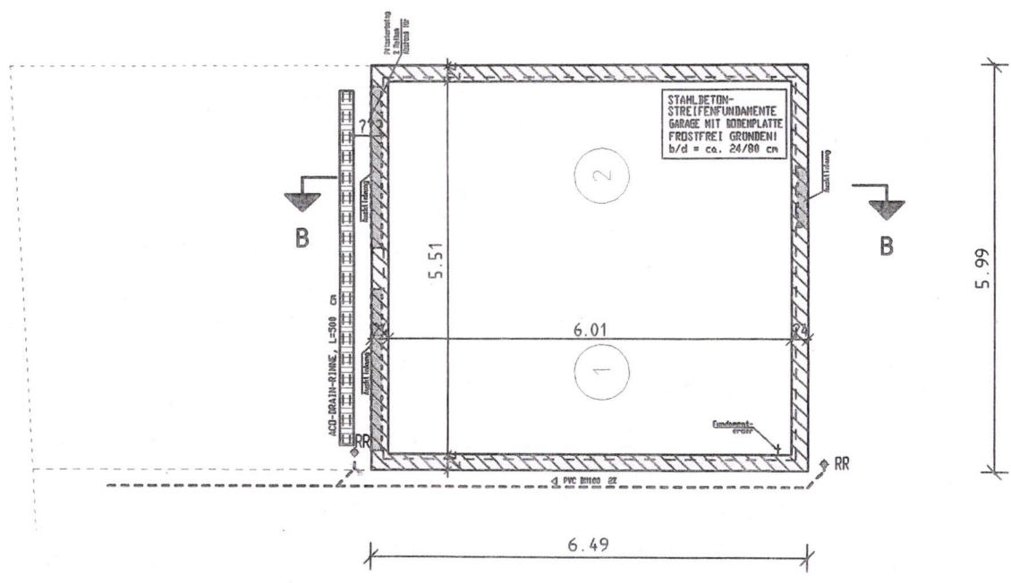
FUNDAMENTE
