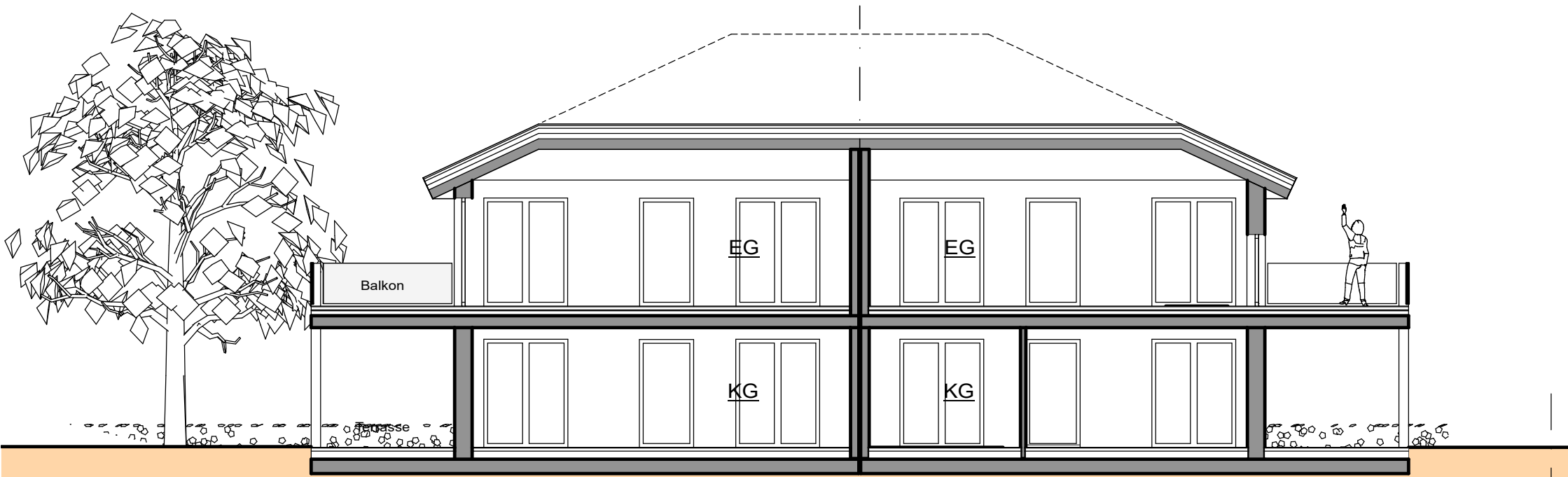
SCHNITT: A - A
