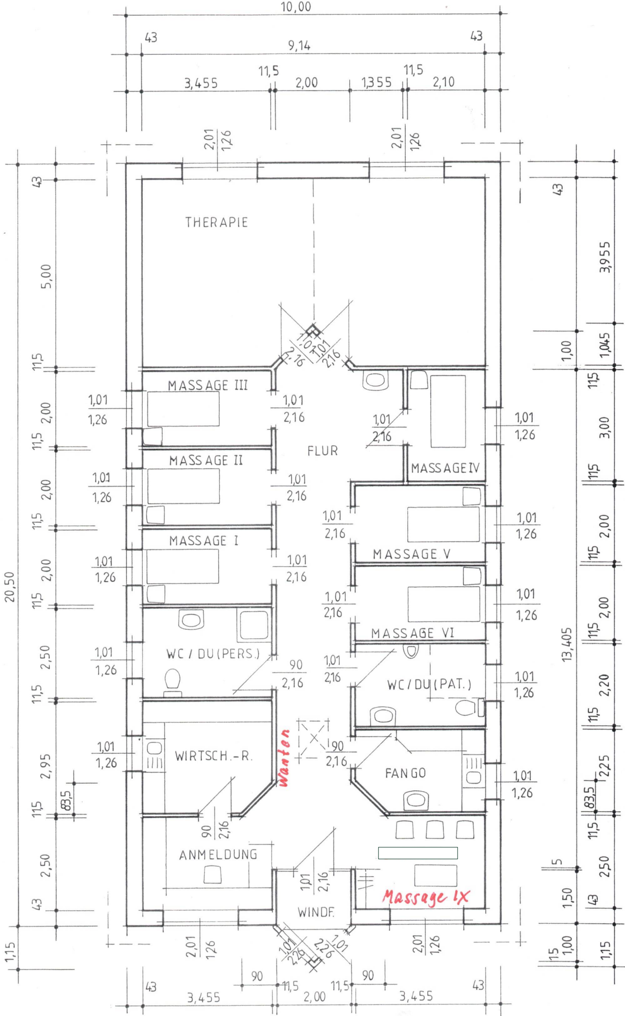
GRUNDRISS
