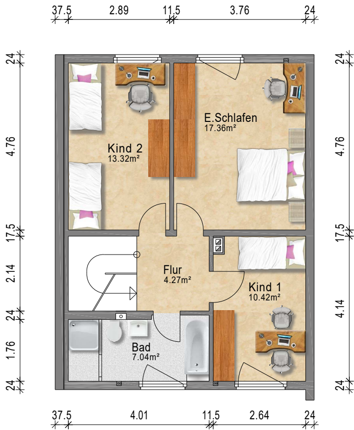
Obergeschoss
