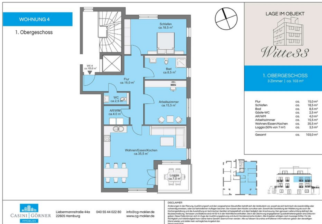
Grundriss WE4
