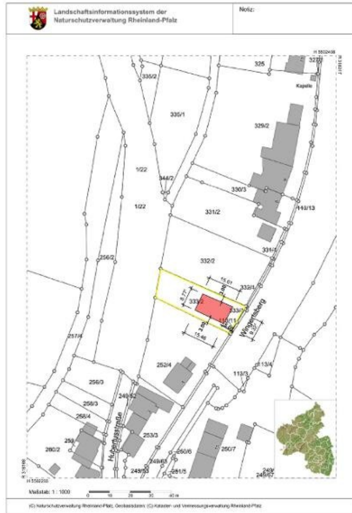
Lageplan
