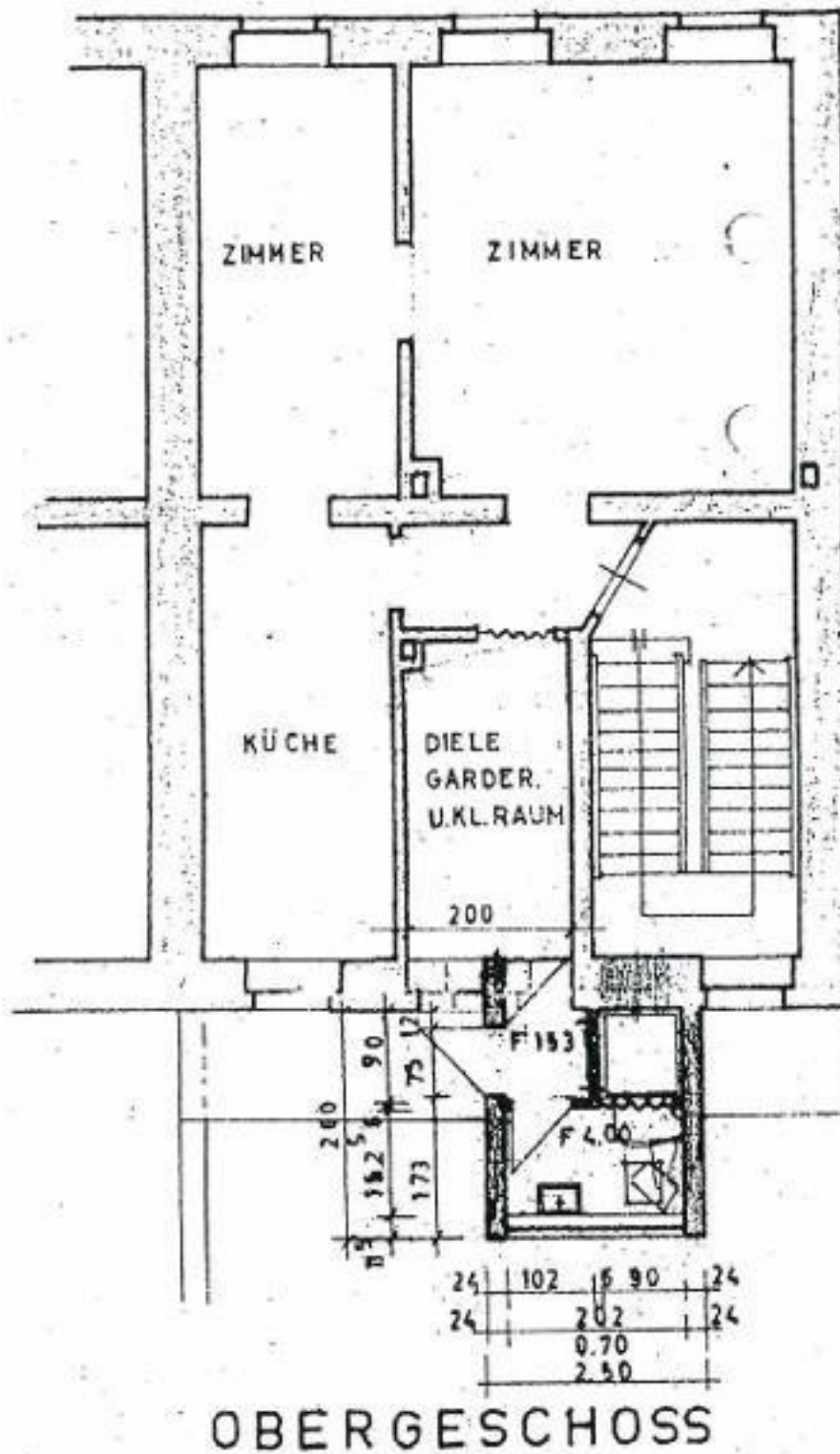
Grundriss
