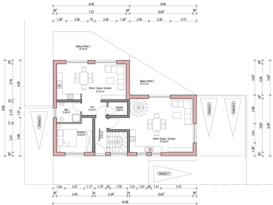
Grundriss Erdgeschoss
