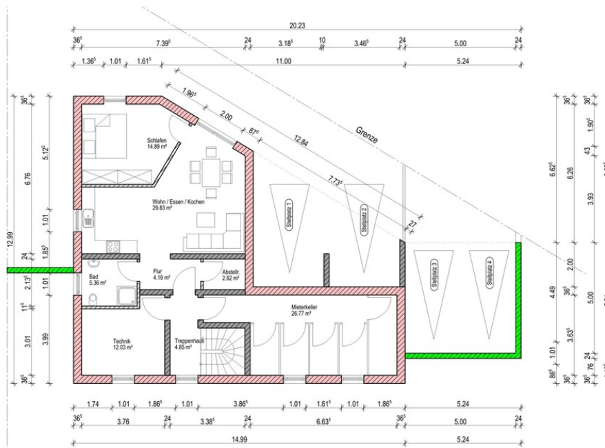
Grundriss Untergeschoss
