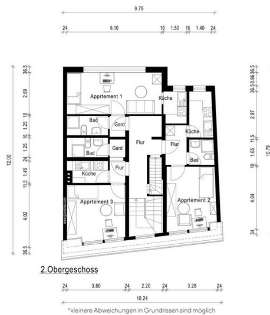
Grundriss 2. Obergeschoss
